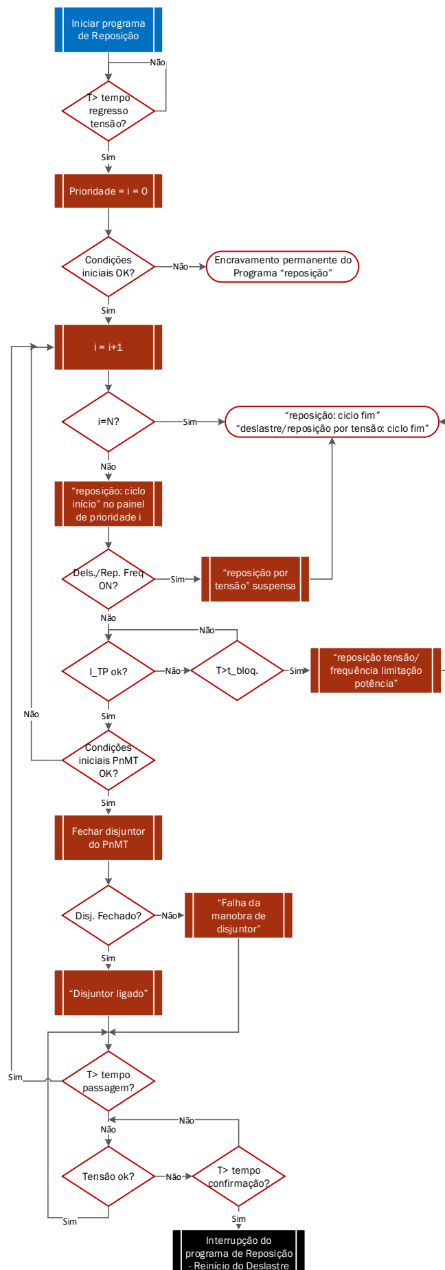
Figura 4.2 - Fluxograma do automatismo Deslastre/Reposição de tensão - Reposição
