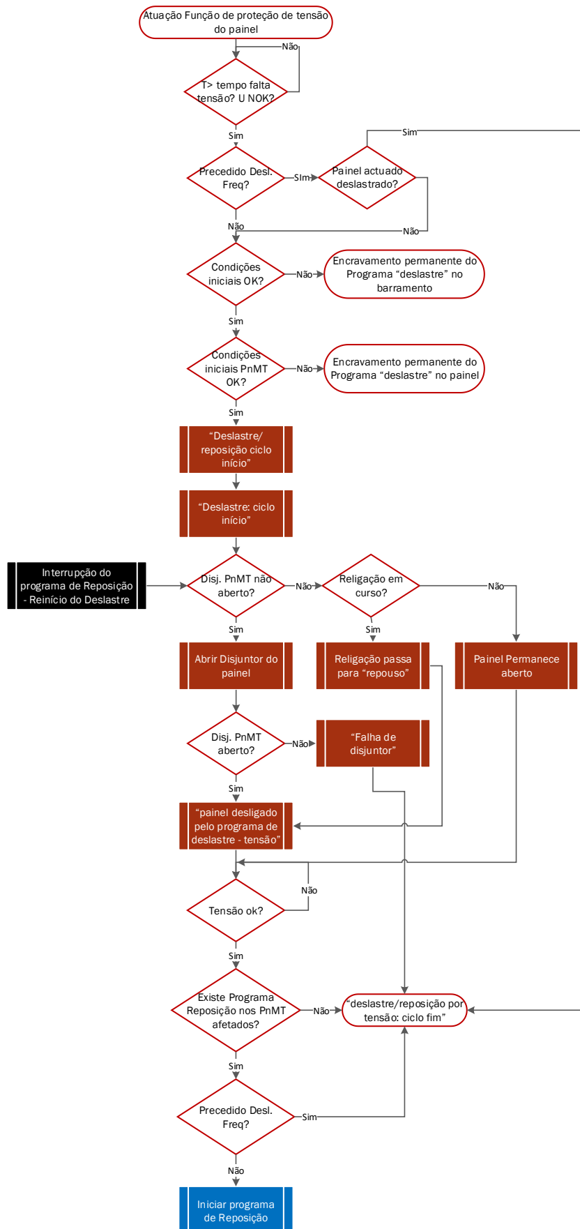
Figura 4.1 - Fluxograma do automatismo Deslastre/Reposição de tensão - Deslastre
